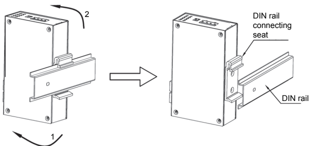
Figure 6 DIN Rail Dismounting
