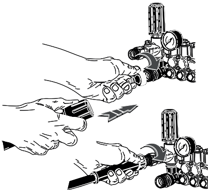
Vesikytkentä.
