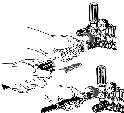
Wateraansluiting.
