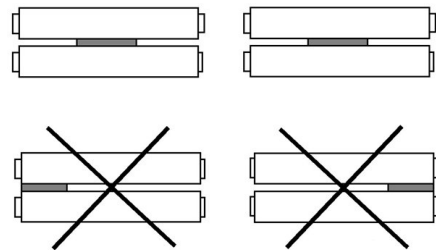
Abb. 11: Werkstück in der Mitte der Walzen positionieren
