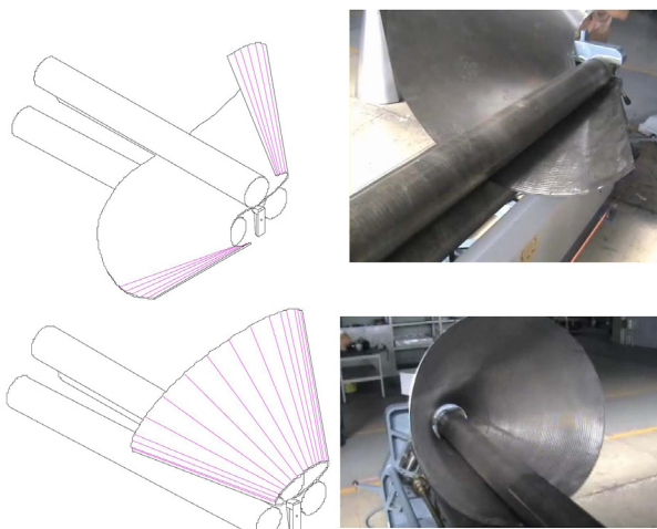
Abb. 18: Konisch Biegen, Ablauf
