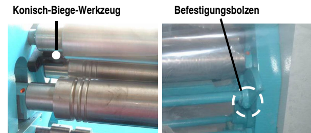
Abb. 16: Konisch Biegen: Werkzeug (links) und Bolzen (rechts)
