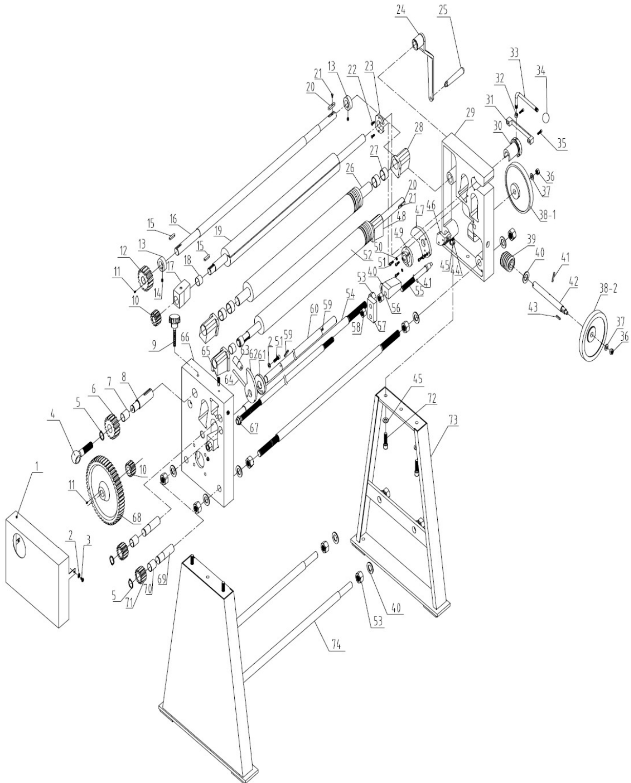
Abb. 22: Ersatzteilzeichnung RBM 1000-20 ECO
