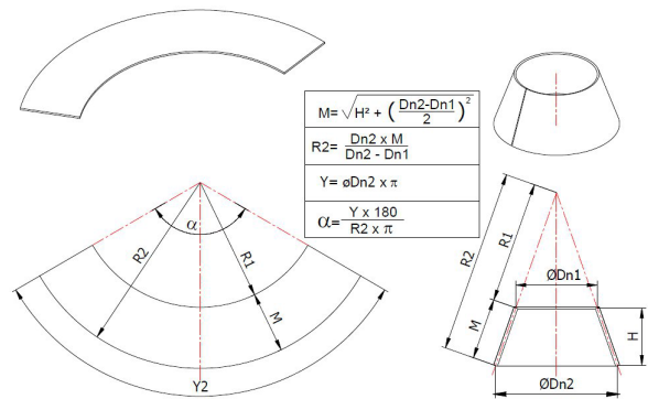
Abb. 15: Berechnung der Werkstückmaße
