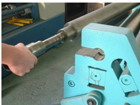
Abb. 19: Oberwalze schwenken
