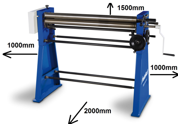
Abb. 6: Arbeitsbereich an der Maschine
