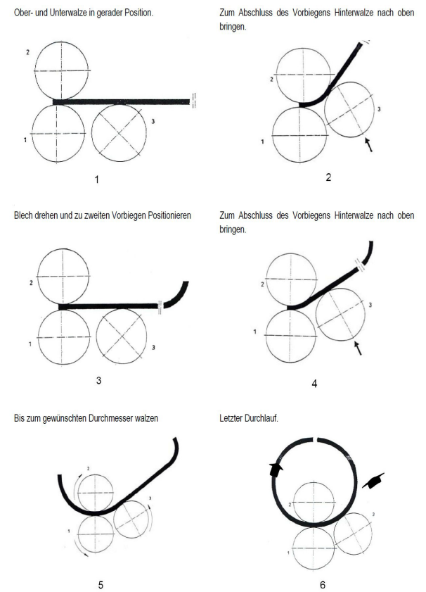
Abb. 14: Biegevorgang
