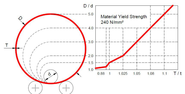
Abb. 13: Biegediagramm
