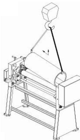
Abb. 20: Werkstück-Entnahme mit Hebevorrichtung
