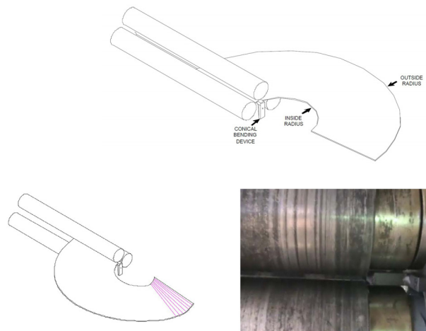
Abb. 17: Konisch Biegen, Vorbereitung
