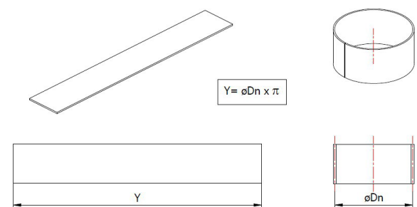
Abb. 12: Berechnung der Werkstücklänge
