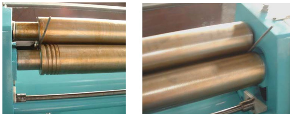
Abb. 10: Parallelität der Walzen prüfen
