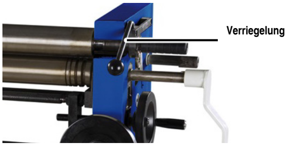
Abb. 9: Verriegelung der Oberwalze lösen
