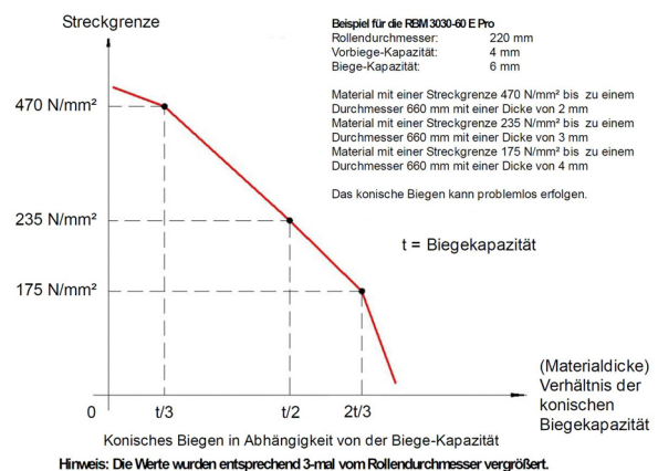
Abb. 3: Diagramm für Streckgrenzen
