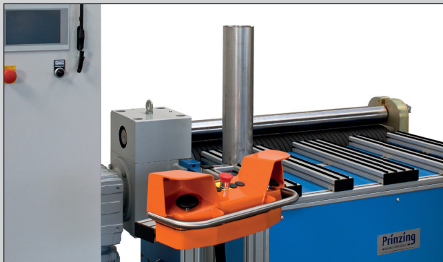
Zweihandbedienung / Two hand switch
