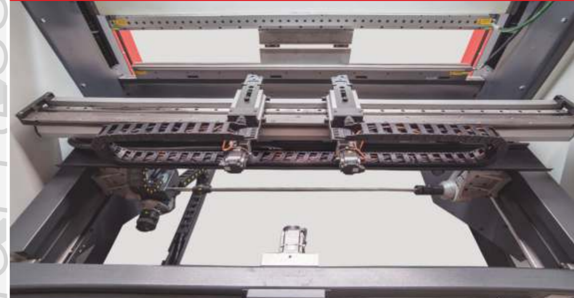
X - R - Z1 - Z2 4 AXIS BACK GAUGE OPTION
