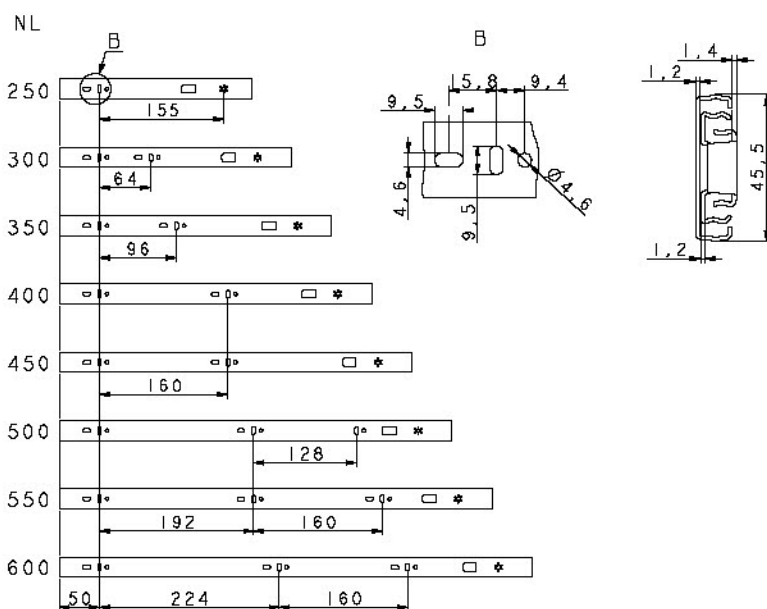
NL - DŁUGOŚĆ NOMINALNA / NOMINAL LENGTH
