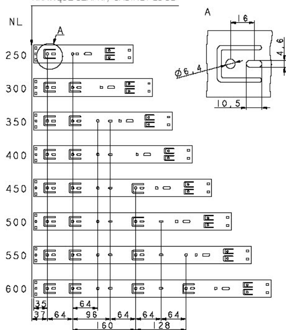
KRAWĘDŹ SZAFKI / CABINET EDGE
