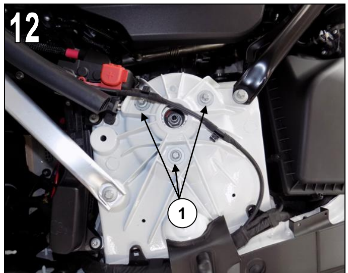
Abb. 12 Schrauben (1) des Stützlagere lösen. Federbein gegen Herabfallen sichern.
