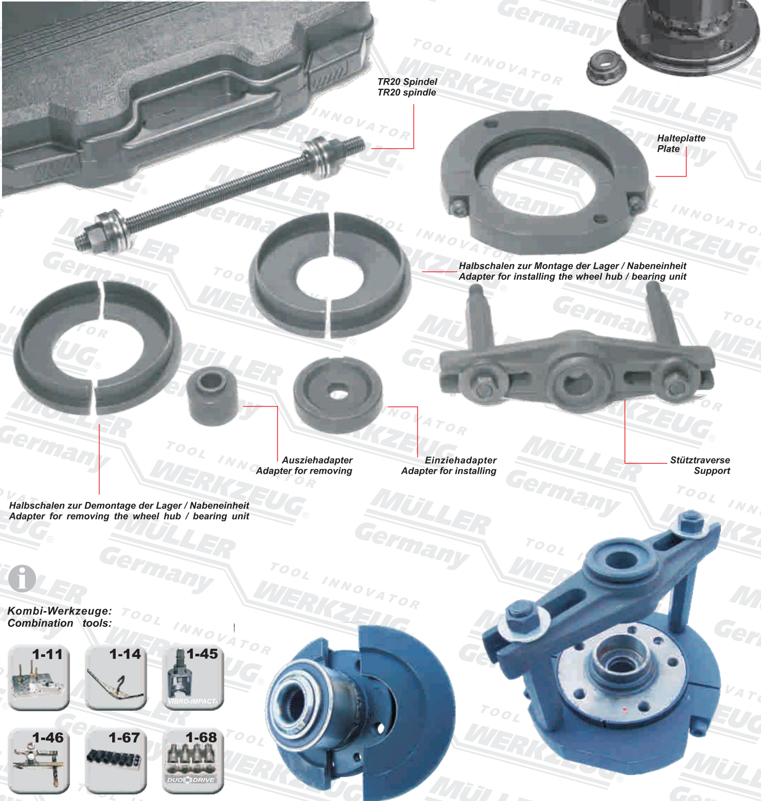
VW T5 Lager / Nabeneinheit VW T5 wheel hub / bearing unit
