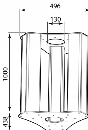
Takfäste
