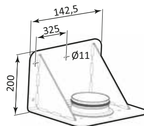
Väggfäste
