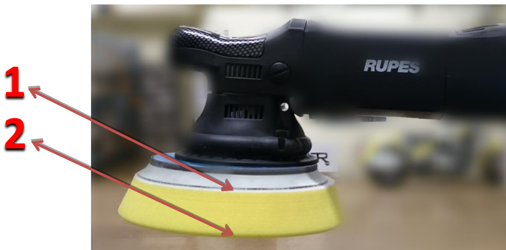
Friktionsvärme skapas i zon 1 och 2
