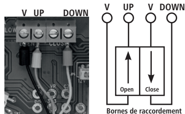
Bornes de raccordement pour bouton-poussoir externe
