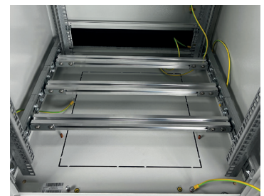
09AA H2000xB600xD600mm med en batterihylla & standard 42U rackskenor
