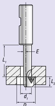
BV, Cajeado inverso
