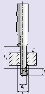
DFV 90°, Achaflanado frontal/inverso
