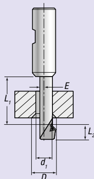
BFV 90°, Achaflanado inverso
