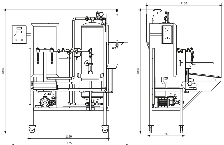
Halbautomatische Bag in Box Abfüllanlage
