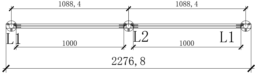
(P) PLAN 2 SCALE: 1:1
