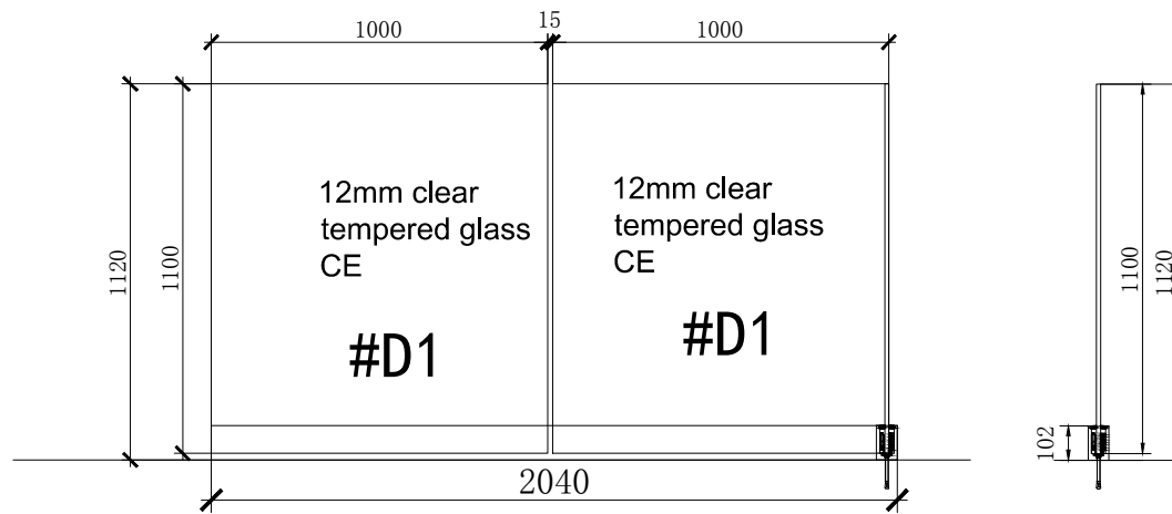
EL 10B-ELEVATION SCALE: 1:1
