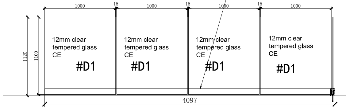
EL 2A-ELEVATION SCALE: 1:1
