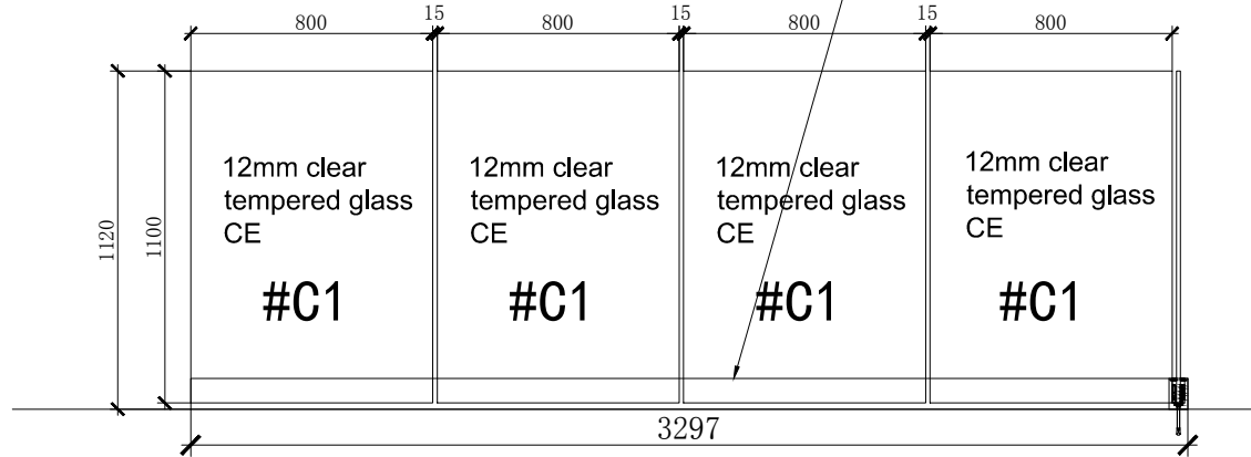
EL 9A-ELEVATION SCALE: 1:1
