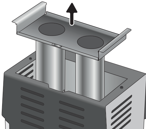
Abb. 4: Rösteinsatz ausbauen
