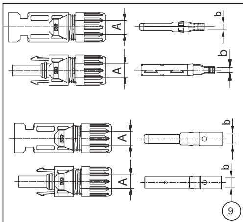
(ill. 9, Tab. 1 + 2) Kontrollieren Sie die Masse A und b gemäss Illustration 9 und Tabelle 1 und 2.
