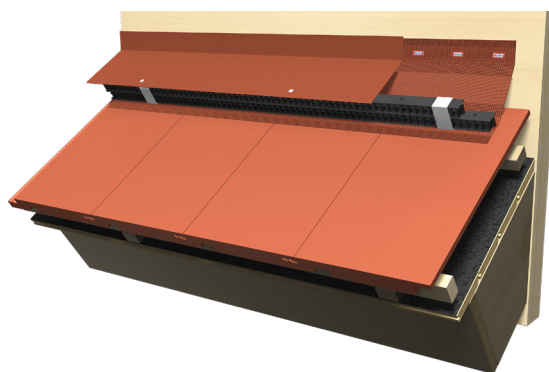
Vägganslutning
