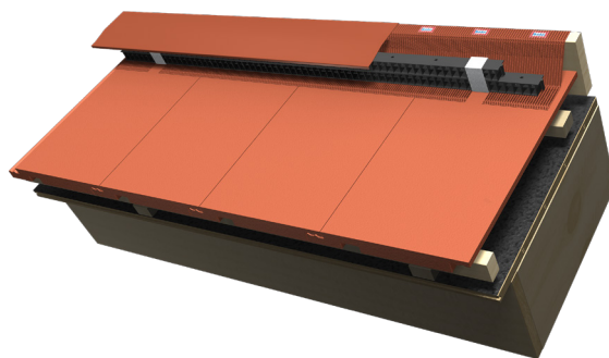
Pultavslut
